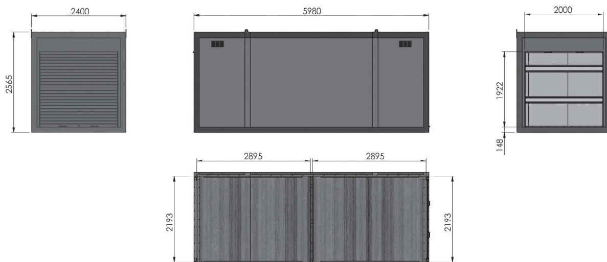
Container compartimenté - Type 1 580 40 002
